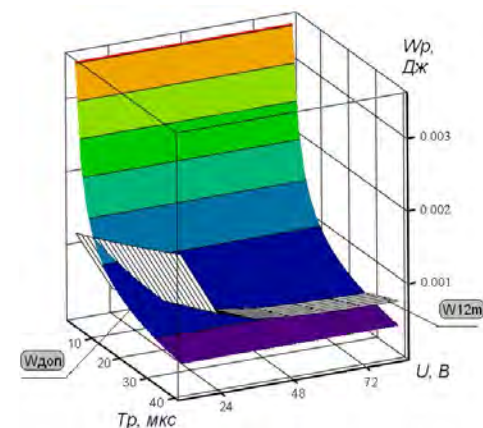
Рис 4 - Зависимости величины максимума энергии разряда ( W_{12m} ) и минимальной допустимой энергии воспламенения ( W_{\text{доп}} ) от напряжение источника питания ( U ) и длительность разряда ( T_p ) для технологической среды метановоздушная смесь
