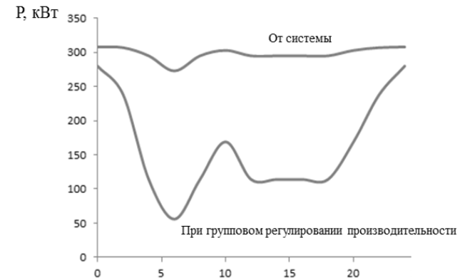
Рис. 2 – Потребление электроэнергии механизмами тяго-дутьевой системы котла
