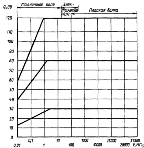
Рис. 1. - Зависимость эффективности экранирования ЭК от частоты
