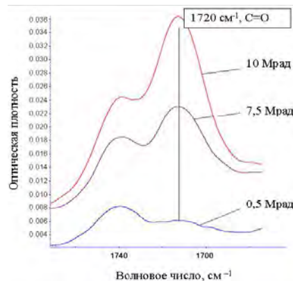
Рис.3 - Зростання оптичної густини смуги 1720 \text{cm}^{-1} в опромінену поліетилені зі збільшенням поглиненої дози
