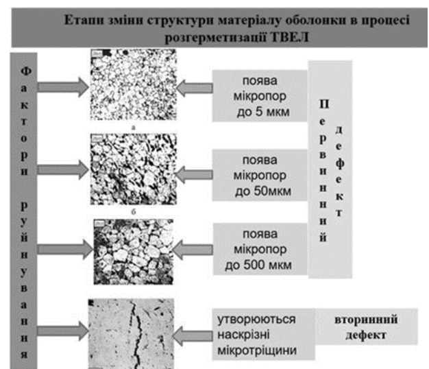
Рисунок 1 – Процес утворення первинних і вторинних дефектів при пошкодженості структури матеріалу оболонки ТВЕЛ
